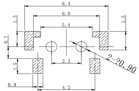
P.C.B 板焊接图
